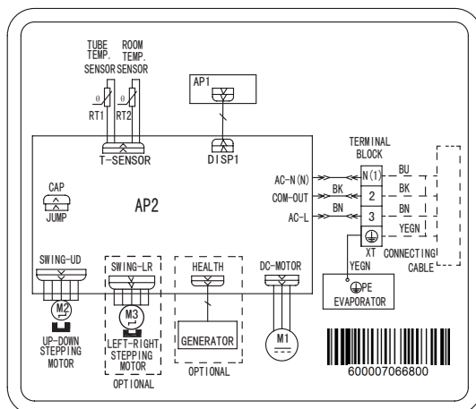
Sisäyksikön kytkentätäulu
