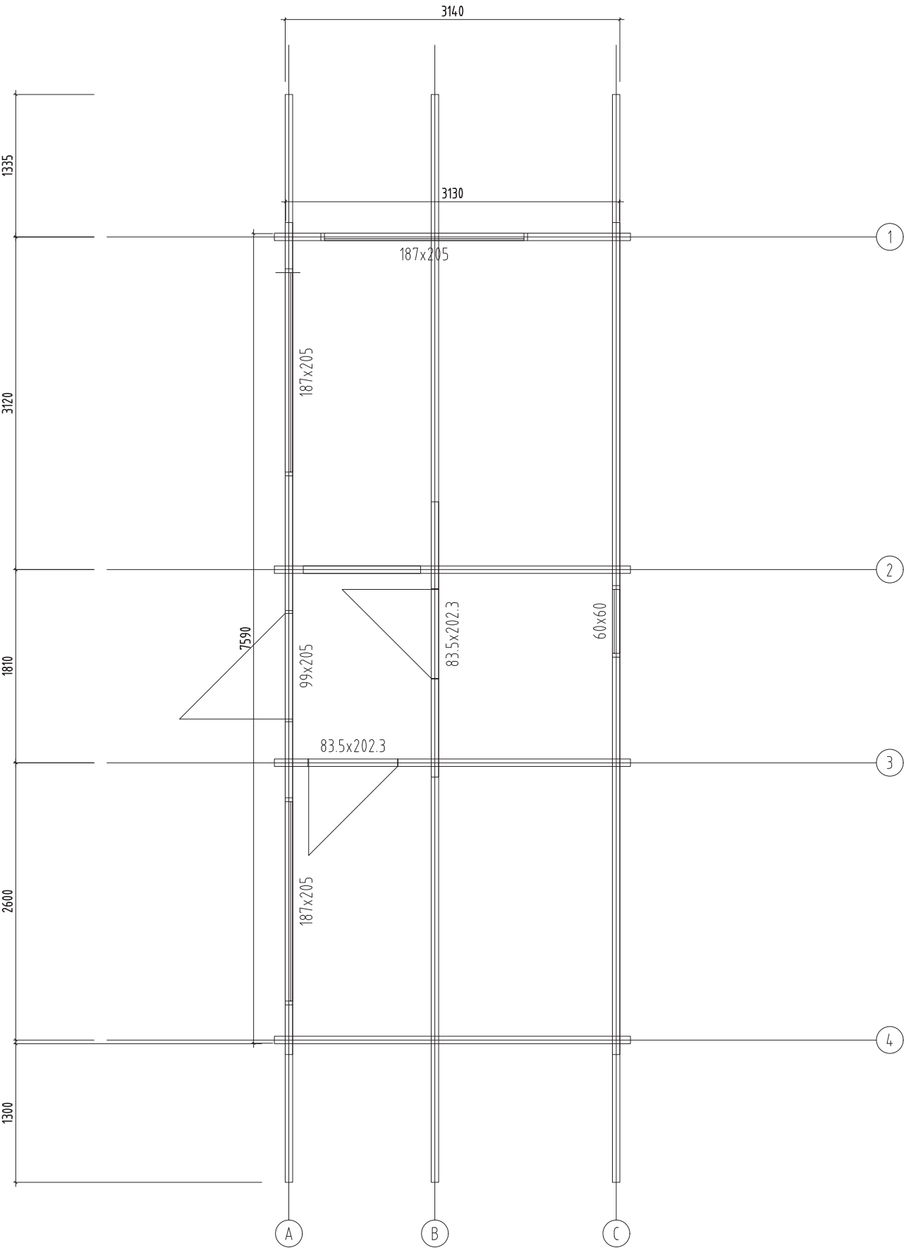
Plan 2 : Wall plan
